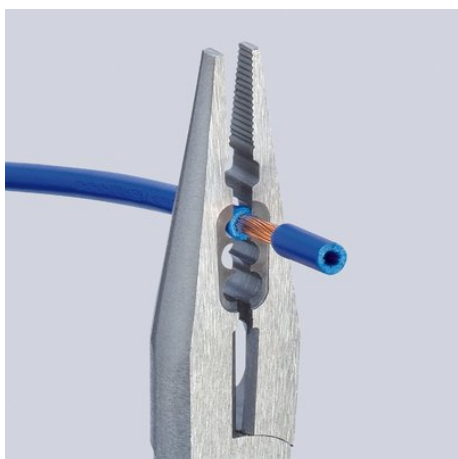
Зачистка 0,5 - 0,75 / 1,5 / 2,5 мм 2
